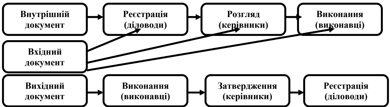
Рис.1. Схема документообігу
